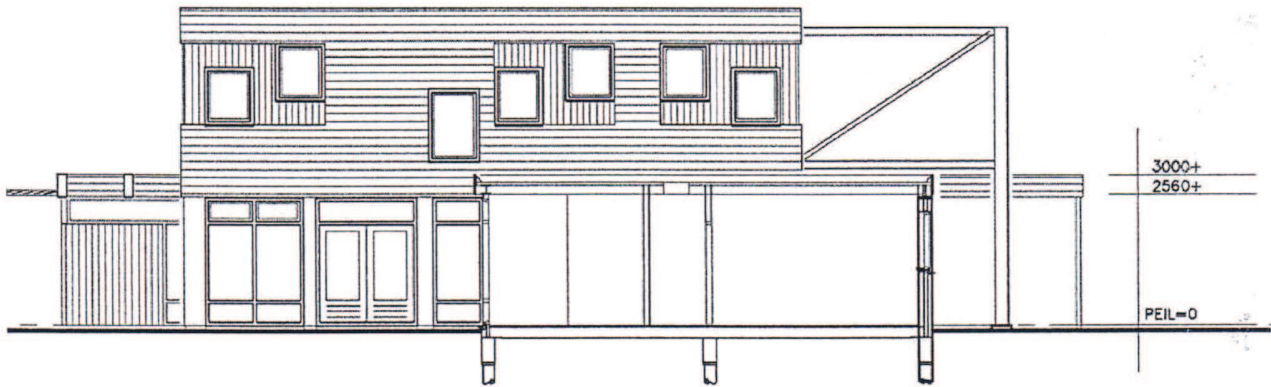
doorsnede A-A
